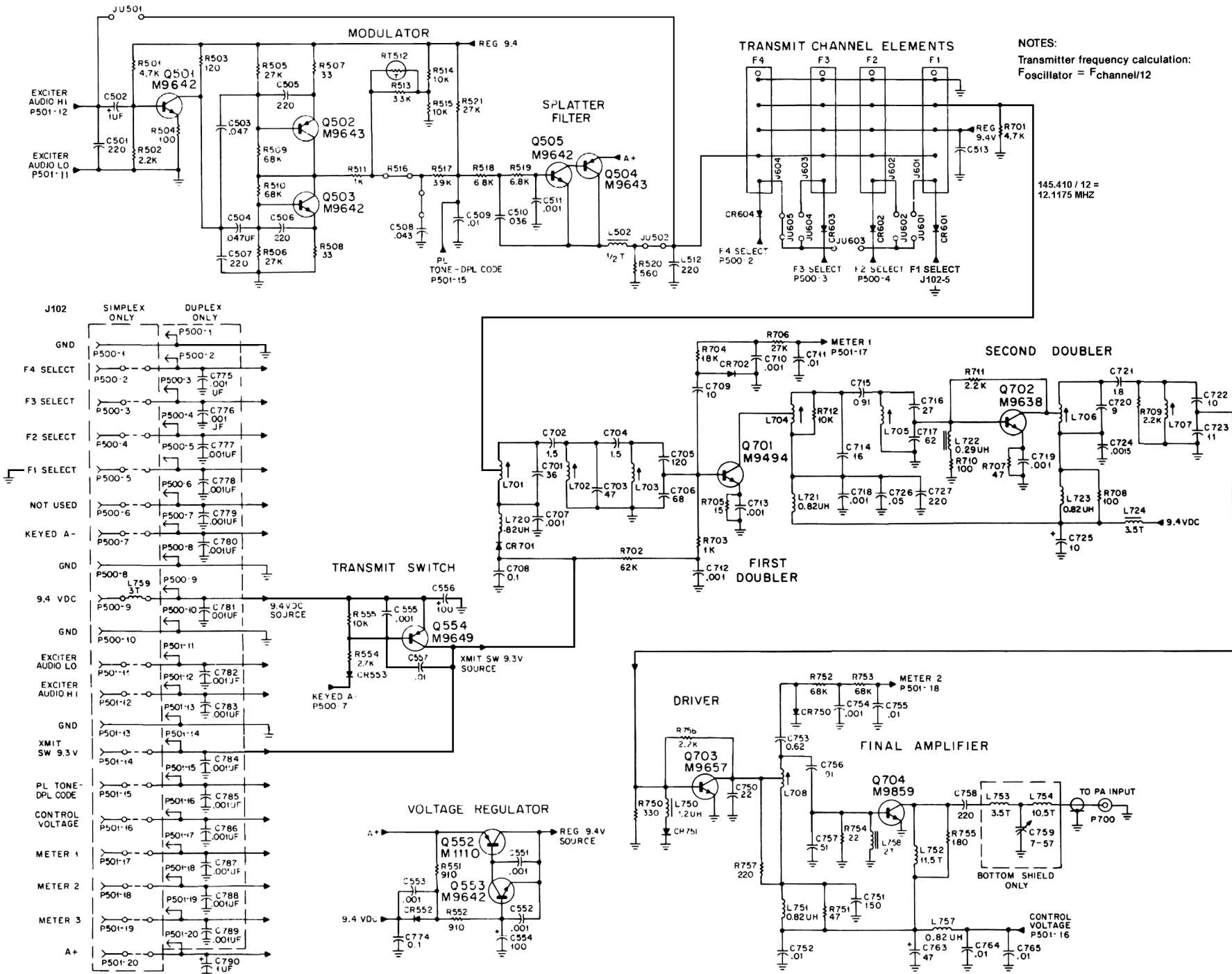
Exciter - TLD9232B
